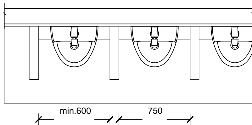
Urinal( Plan)
