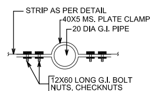
DETAIL-A (SCALE-N.T.S.)
